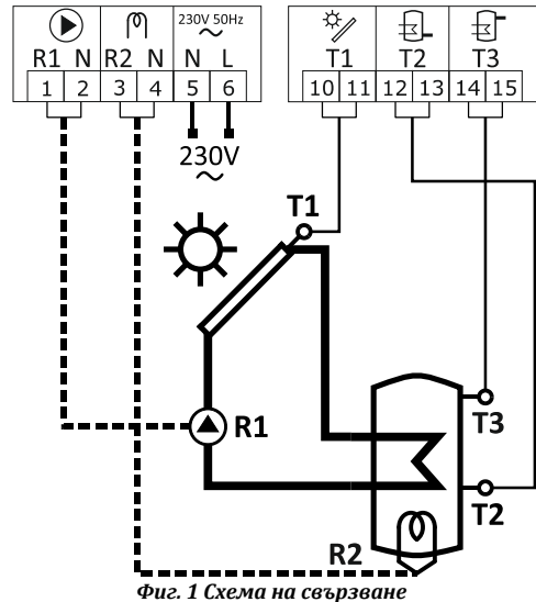
Фиг. 1 Схема на свързване
